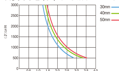
スリップジョイント S2 (面材厚さ 0.3mm)
