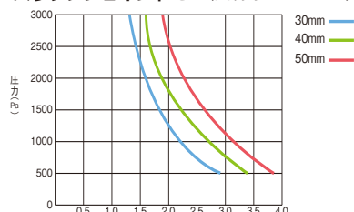
スリップジョイント S2 (面材厚さ 0.35mm)
