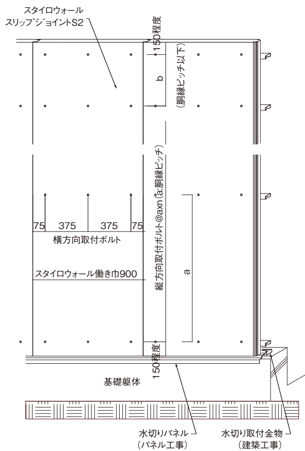
外部立面図
