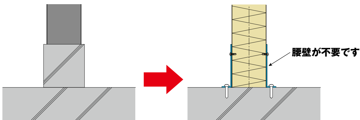
ALCパネルの場合
